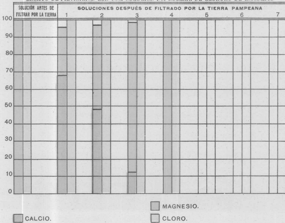
ENSAYO DE FILTRACIÓN CON UNA SOLUCIÓN 1/10 NORMAL DE CLORURO DE MAGNESIO
