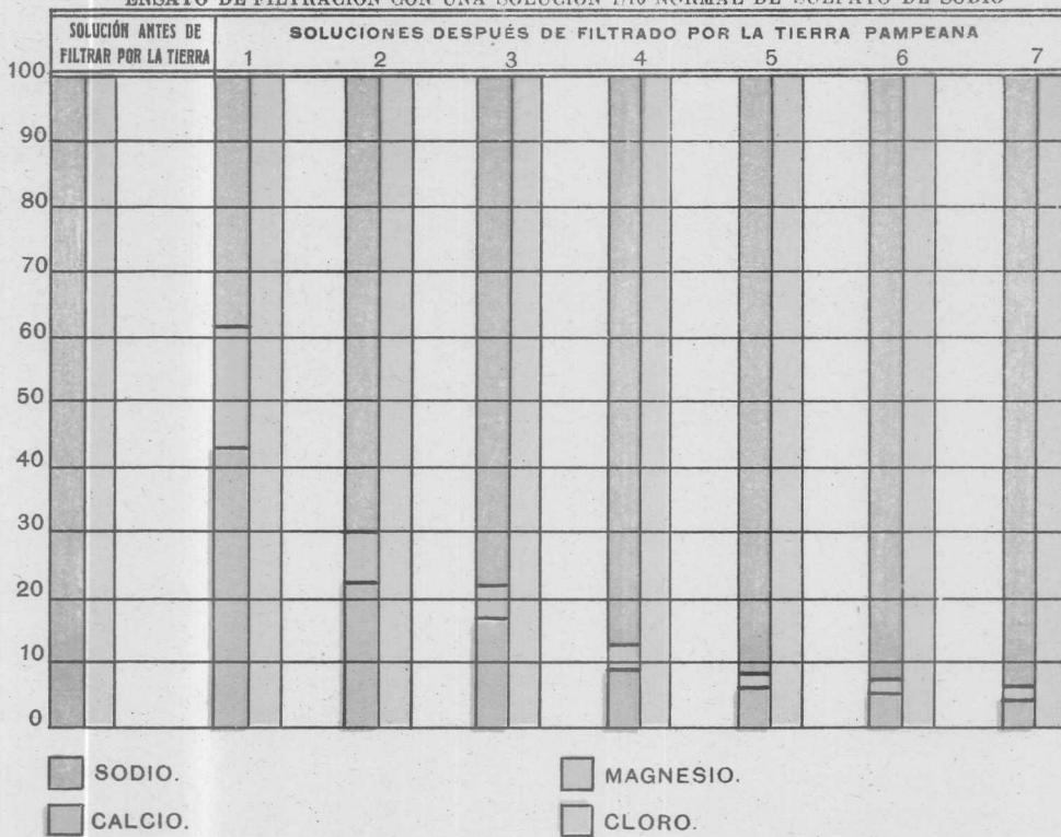
ENSAYO DE FILTRACIÓN CON UNA SOLUCIÓN 1/10 NORMAL DE SULFATO DE SODIO
