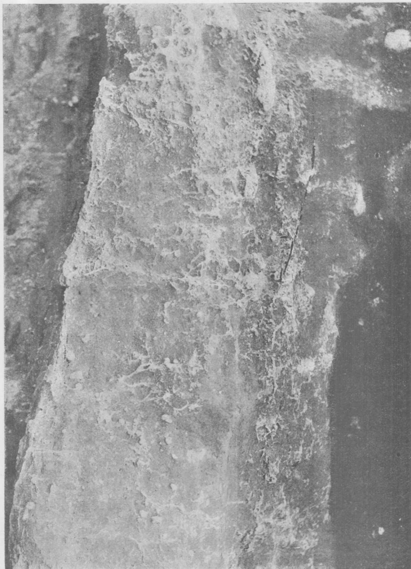
Fig. 17. — Estructura de capa lacustre del horizonte mesopampeano, intercalada en el loess
