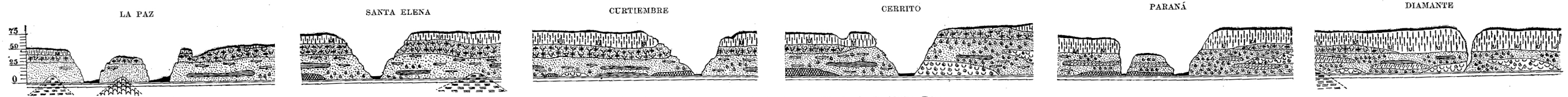
Perfil de las barrancas del río Paraná, provincia de Entre Ríos
