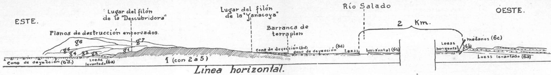
Fig. 31. — Perfil general de Mazán. Escala 1 : 50.000
