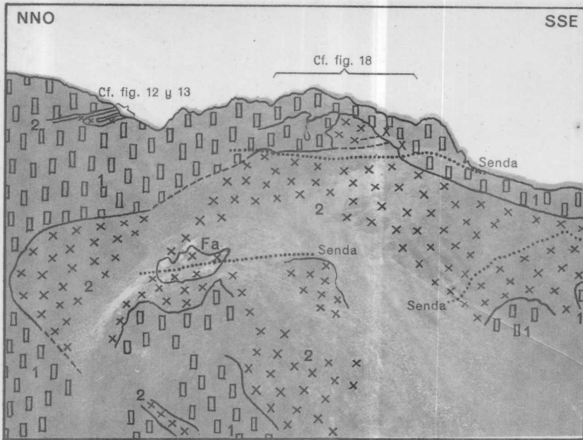
Fig. 16. Sobreescorrimiento del granito antiguo sobre el joven. Mazán
