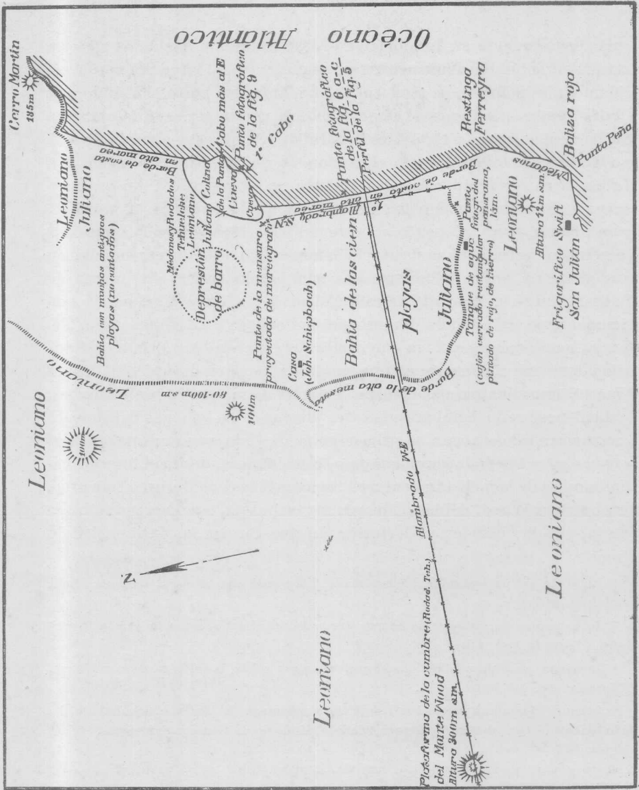
Fig. 4. — Croquis geo-morfológico de la región entre Punta Peña, el Cabo Curioso y Monte Wood, entre 7 a 16 kilómetros al NNE y 7 kilómetros al NNW respectivamente de San Julián. Escala 1 : 50000
