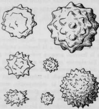
Fig. 18. — Microscleras de Esponjas del « banco verde » de paso Niemann, 600 : 1
