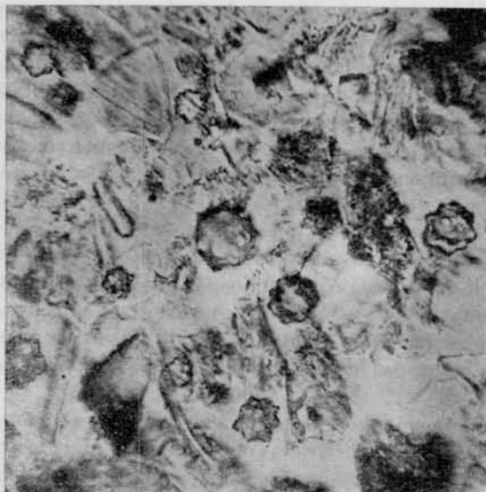
Fig. 16 — Microscleras de Spongillidae en los tobos del Casamayorenses del Cañadón Féola (Chubut)
