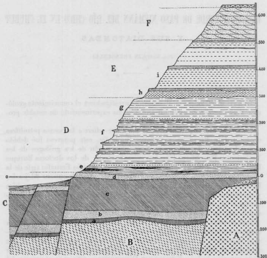
Fig. 1. — Serie estratigráfica normal en proximidad del borde septentrional de la cuenca petrolífera de Comodoro Rivadavia, Chubut (perfil esquemático) : A, Pórfido cuarcífero y rocas asociadas; B, Pehuenchiano; C, Salamancaiano : a, « lignífero », b, « glauconítico », c, « fragmentoso », d, « banco verde » = Salamancaquense; D, Deseadiano : e, basal con « bancos negros », f, Riochiquense, g, Casamayorens-Deseadense; E, Patagoniano : h, Juliense, i, Leonense, j, Superpatagoniense; F, Entrerriano; G, Tehuelchiano.
