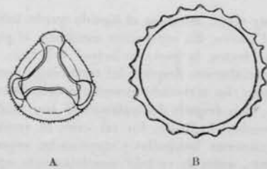
Fig. 19. — A, Thraanium sp.; B, Metocena circularis Ehr. 600 : 1
