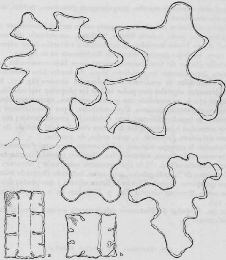
Fig. 17. — Células silíceas de Gramináceas del « banco verde » de paso Niemann, 600 : 1
