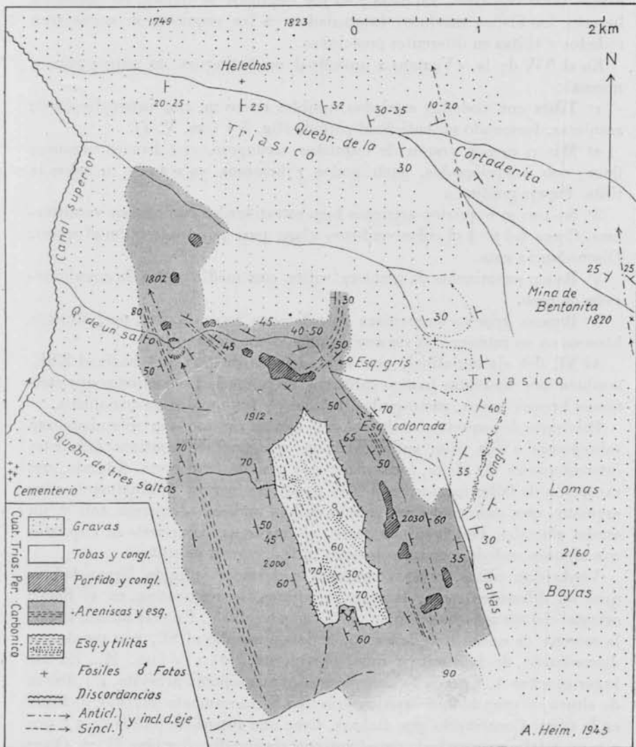
Fig. 1. — Parte norte de la Sierra del Barreal. Croquis tectónico 1 : 40.000, a base del mapa 1 : 50.000 del Instituto Geográfico Militar, ed. 1935
