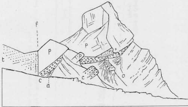
Fig. 8. — Bloque fracturado de pórfido cuarcífero (p) al lado norte de la quebrada de Un Salto; relicto en un foso de areniscas esquistosas del Carbónico (a). c, conglomerado de base; r, toba morada descompuesta; f, falla?; + falla ondulada con estrías horizontales de rumbo N25W. Vista hacia SE.
