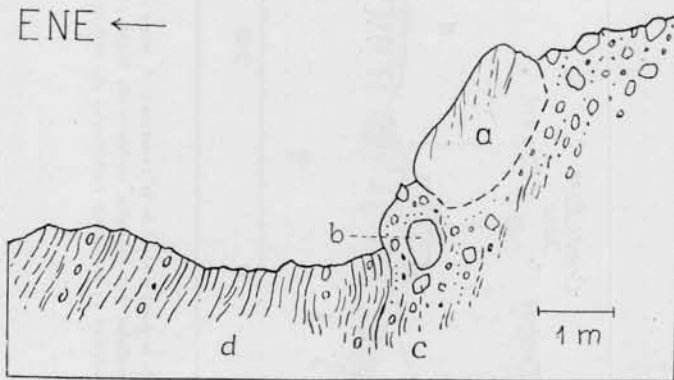
Fig. 3. — Posición tectónica del bloque errático estriado de diabasa (a) en la parte SE de la « ventana » (Véase lám. II, 2); b, bloque redondeado 50 × 75 cm, bien estriado; c, bloque de granito 30 × 25 cm; d, parte basal de unos 80 m de esquistos verduscos, con algunos rodados glaciares estriados.
