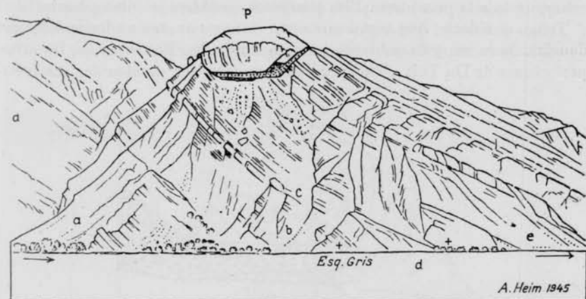
Fig. 6. — La Esquina Gris en la Quebrada de Un Salto (Quebr. d. l. Cerros Colorados). Véase texto
