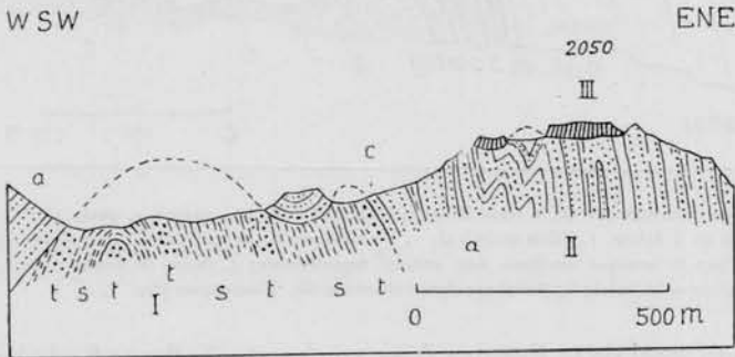
Fig. 4. — Perfil transversal esquemático a través de la parte sur de la « ventana ». I-III como en fig. 2. a, areniscas rojizas y blancas; c, conglomerado de base; s, esquistos verduscos; t, tilitas
