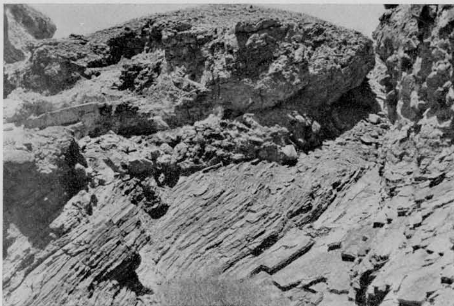
1. Detalle del pórfido cuarcífero sobre el Carbónico (areniscas esquistosas). Entre ambos el conglomerado grueso de base. Lugar al lado del bloque de la figura 8 del texto
