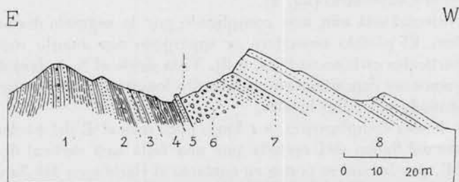
Fig. 10. — Contacto de la serie carbónica 1-5 con la tilita, 150 m al ESE de la casa Leoncito Encima. 1, Esquistos verduscos con bancos de grauvaca gruesa, intercalada por esquistos; 2, 3-5 m arcillas verduscas arenosas; 3, 6-8 m bancos de grauvaca gruesa intercalada por esquistos de grauvaca calcárea en la parte inferior; 4, 1-3 m arenisca (grauvaca) micécea con restos de plantas, inclinada 65° hacia W 30°N. Se destaca el banco superior de 30 cm con su superficie estriada por el glaciar carbónico. (Compárese lám. V, 2); 5, 10-15 m tilita, morena de fondo; 6, 4 m pasaje de morena al conglomerado y la arenisca fluvioglacial; 7, parte basal de más de 50 m de arenisca parda-amarilla, carbónica, inclinada 30-35° hacia W 20° S.
