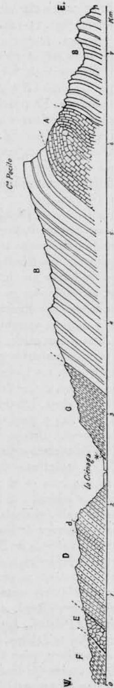
Fig. 10. — Croquis del perfil de la Sierra de Huaco : A, Ordovícico ; B, Estratos de Guandacol ; C, Estratos de Patquía ; D, Estratos de Patquía ; E, Aglomerado porfirítico dislocado del Cenoico ; F, Rodados dislocados del Cenoico ; d, nivel calcífero de los Estratos de Patquía ; * Yacimiento fosilífero de los Estratos del Tupe
