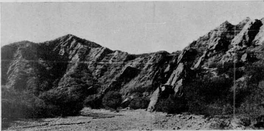
Fig. 3. — Quebrada de la Higuera. Rodados dislocados del Cenozoico (a la izquierda) en aparente concordancia con los Estratos de Patuía (a la derecha)
