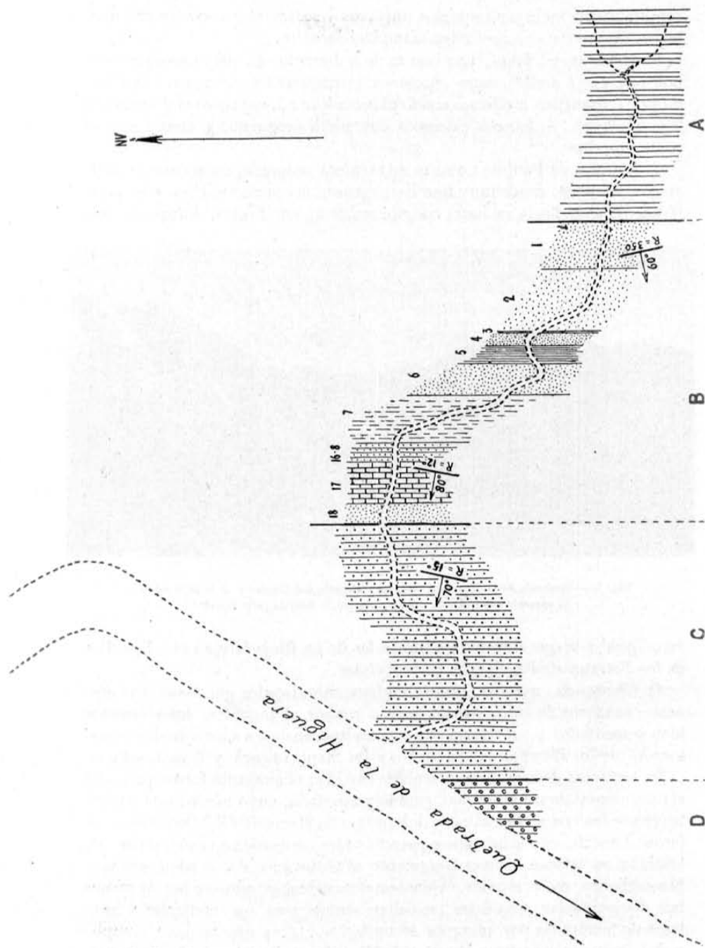
Fig. 4. — Croquis geológico de la Quebrada de la Herradura : A, Estratos de Guandacol ; B, Estratos del Tupu ; C, Estratos de Pastoquia ; D, Rodados dislocados del Cenozoico. Escala 1 : 3500
