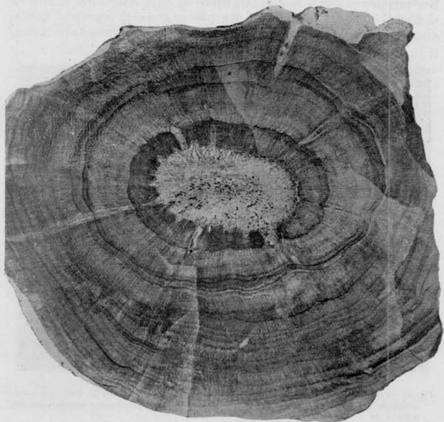
Fig. 24. — Diloxylon sp. con anillos anuales completos del glaci-lacustre del Cerro Colorado de La Antigua. Corte transversal \times 3
