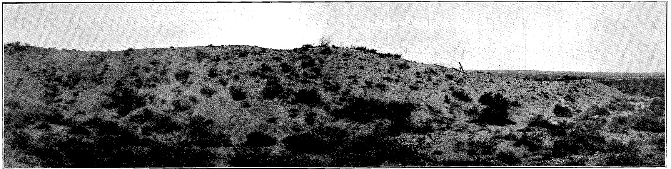
Fig. 2. — Perfil natural del piso Rocanense, 15 kilómetros al norte de Roca (Río Negro)
