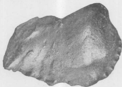
Fig. 2. — Trigonia ? sp. (« Venericardia Ameghinorum » v. Iher.). \frac{1}{4} . Molde, visto hacia la valva derecha. Rocanense intermedio.
