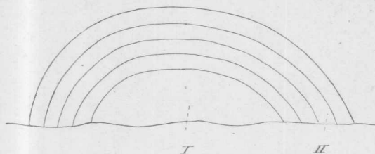
Fig. 1. — Corte esquemático de las capas de caliza porosa pareídas a « Glyptodontia » (? algas calcáreas ?). Al rededor de \frac{1}{2} . Rocanense superior.
