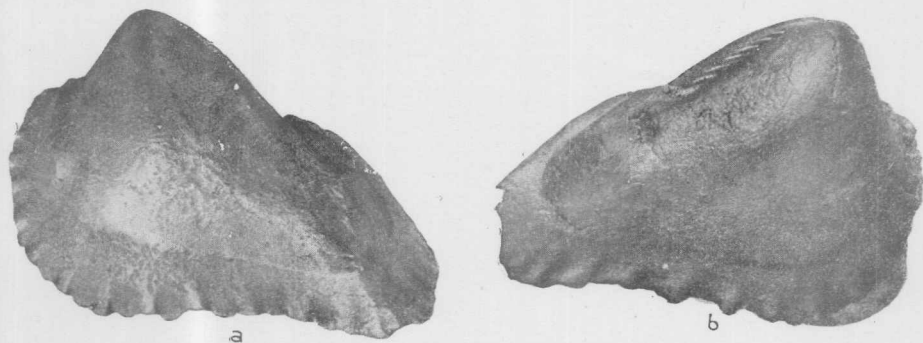
Fig. 1 a-b. — Trigonia ? sp. (« Venericardia [ Cardita ] Ameghinorum » v. Iher.). \frac{1}{4} . Molde, visto hacia la valva izquierda y derecha. Rocanense intermedio
