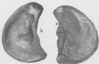
Fig. 4 a-b. — Ostrea Ameghinoi rocana v. Iher. \frac{1}{4} . Valva menor, de afuera y de adentro. Rocanense superior.
