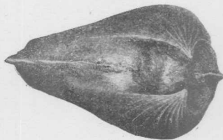
Fig. 3. — Trigonia ? sp. (« Venericardia Ameghinorum » v. Iher.). \frac{1}{4} . Molde, visto de arriba. Rocanense intermedio.
