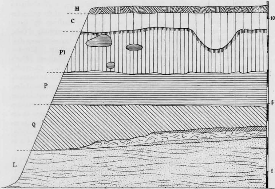
Fig. 3. — Corte artificial para la bajada al puerto de Quequén (1924) : L, Lujanense ; Q, Querandinense ; P, Platense tripoláceo ; PI, Platense loésico (recubierto por costra calcárea) ; C, Cordobense ; H, Humus. Perfil esquemático. (Escala en metros).
