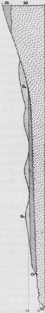
Fig. 1. — Borde del estuario platense en los alrededores de Punta Piedras; E, Ensenadense; B, Bonaerense; Q, Querandinesense; P, Cordones cóncavos del Platense (recubiertos de humus y de monte de Tala); 1, nivel de baja marea; 2, de alta marea. Perfil esquemático.
